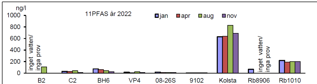
Figur 19 - Summahalten av 11 PFAS i nio grundvattenstationer vid Arlanda flygplats.
